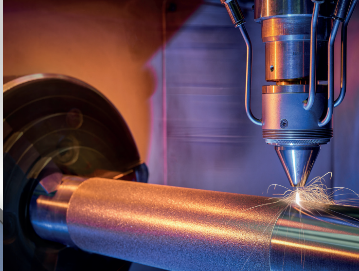
超高速レーザー材料堆積 (EHLA) (© Fraunhofer ILT)
