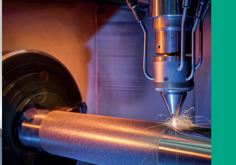
超高速レーザー材料堆積 (EHLA) (© Fraunhofer ILT)
